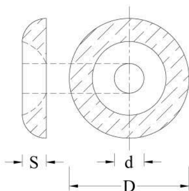
Rondella Cod. 020 Washer No. 020
